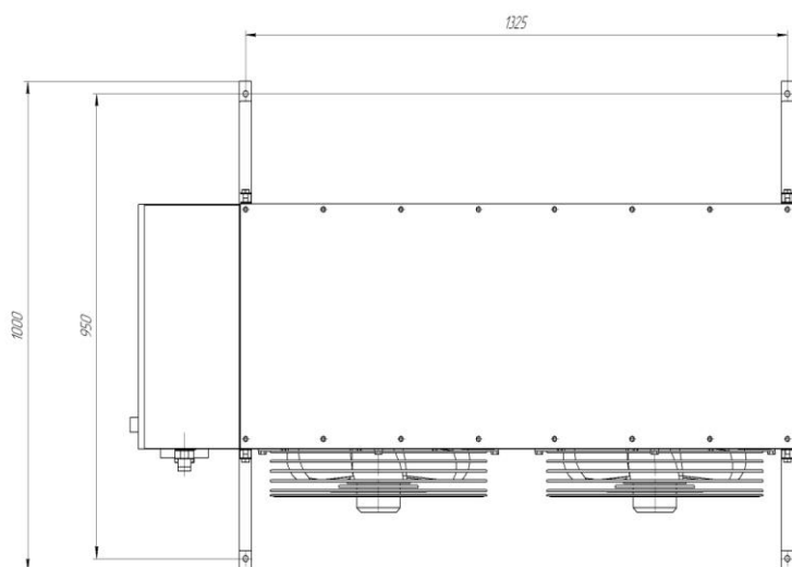
Газификатор углекислотный атмосферный ГУ-500А
