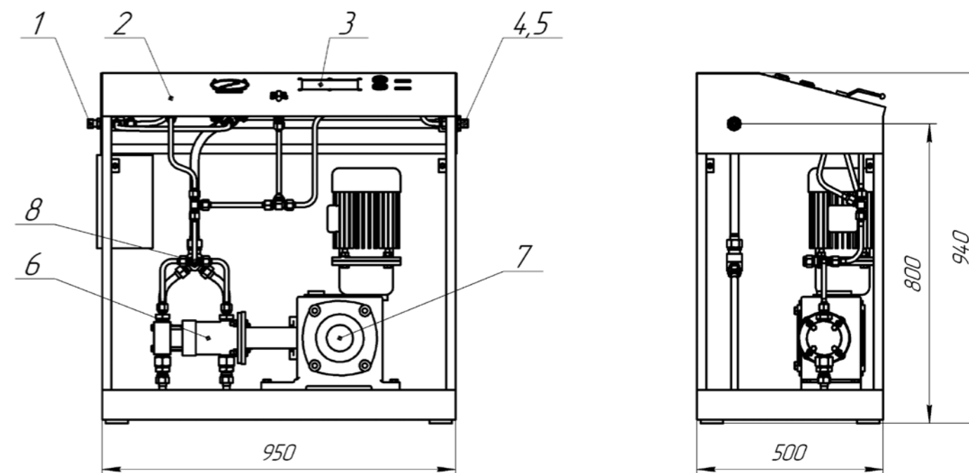
Станция зарядная углекислотная CZY-800 (CZY-800Д). Габаритный чертеж.
